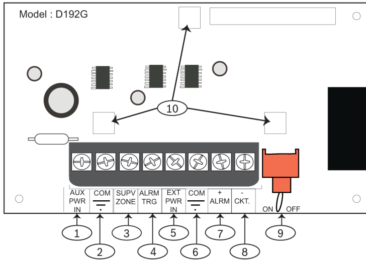
Figure 2.1: D192G_NAC_Module
